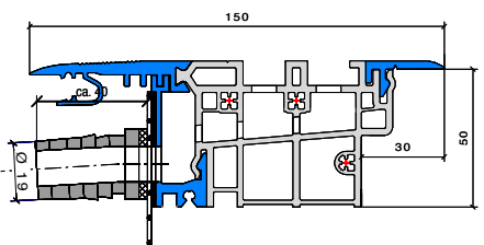
MFAT 10/2 PH mit 50 mm Bodeneinstand
