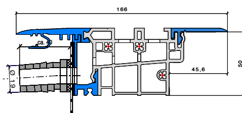
MFAT 10/2a PH mit 50 mm Bodeneinstand
