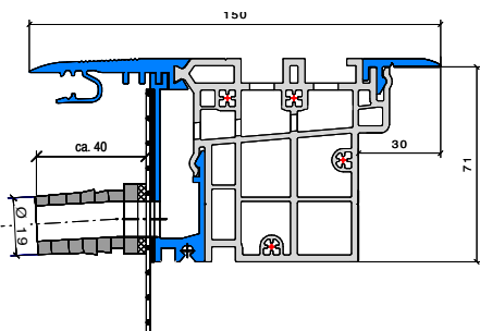
MFAT 10 PH Standardausführung mit 71 mm Bodeneinstand
