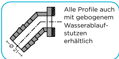
MFAT 10/2a PH mit 50 mm Bodeneinstand
