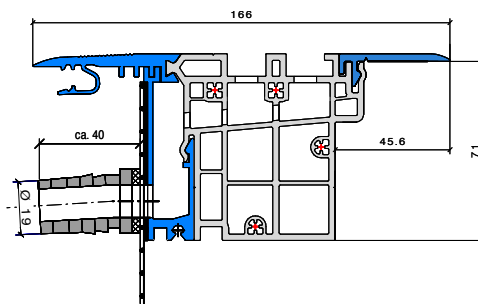
MFAT 10/a PH mit 71 mm Bodeneinstand
